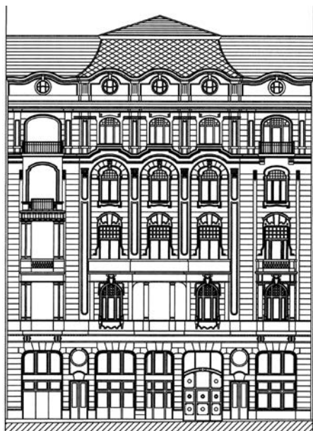
A CSÁKY UTCAI, A ZSINAGÓGÁT IS MAGÁBAN FOGLALÓ BÉRHAZ HOMLOKZATI TERVE
